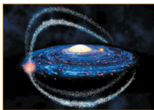
Рис. 2.3. Кільце Єдинорога — протяжний кільцеподібний ланцюг із зір, тричі обернений навколо Чумацького Шляху
