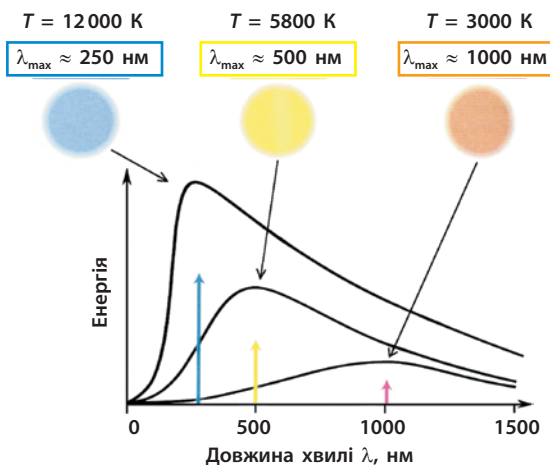
Рис. 1.4. Розподіл енергії у спектрі випромінювання зір. Колір зір визначає температуру поверхні T : сині зорі мають температуру 12 000 К, червоні — 3000 К. При збільшенні температури на поверхні зір зменшується довжина хвилі \lambda_{\text{max}} , яка відповідає максимуму енергії випромінювання
