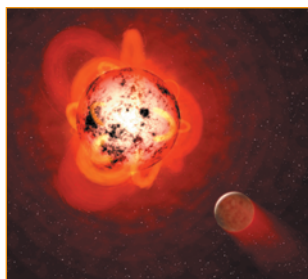
Рис. 1.14. Червоний карлик
