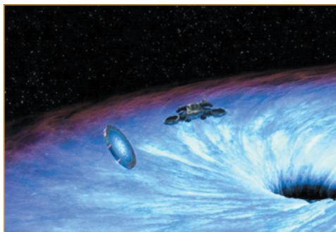
Рис. 3.10. Художнє зображення космічного корабля, що наближається до чорної діри
