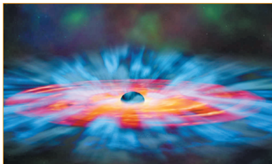
Рис. 3.9. Художнє зображення чорної діри
