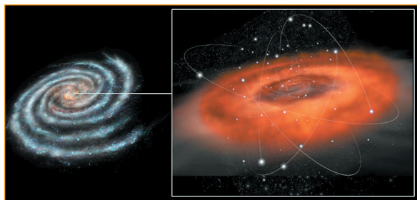
Рис. 2.4. Надмасивна чорна діра Стрілець А*
