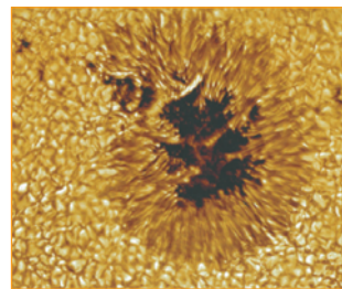
Рис. 3.1. Сонячна пляма — це область фотосфери, де знижується температура, адже сильне магнітне поле у плямі зупиняє конvekцію
