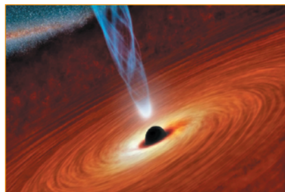
Рис. 2.5. Комп'ютерна модель чорної діри в центрі Галактики
