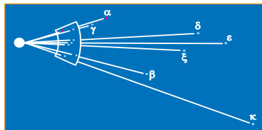
Рис. 1.1. Зорі в сузір'ї Оріон
